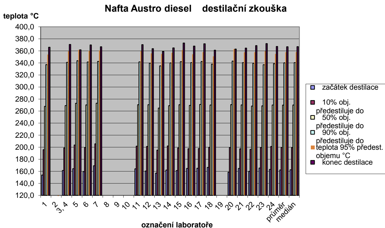
Obr. 4 Destilační zkouška – teplota 95% predest. objemu
