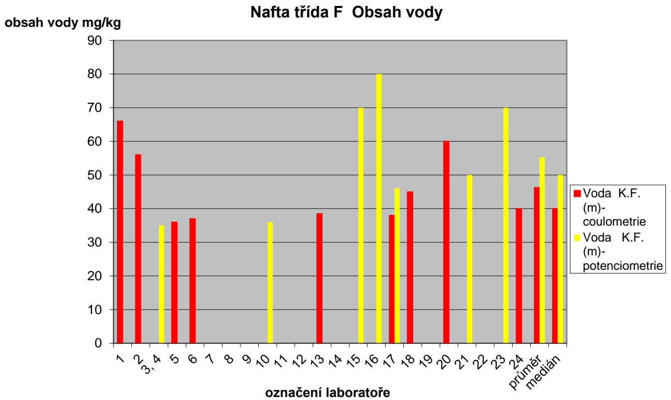
Obr. 17 obsah vody
