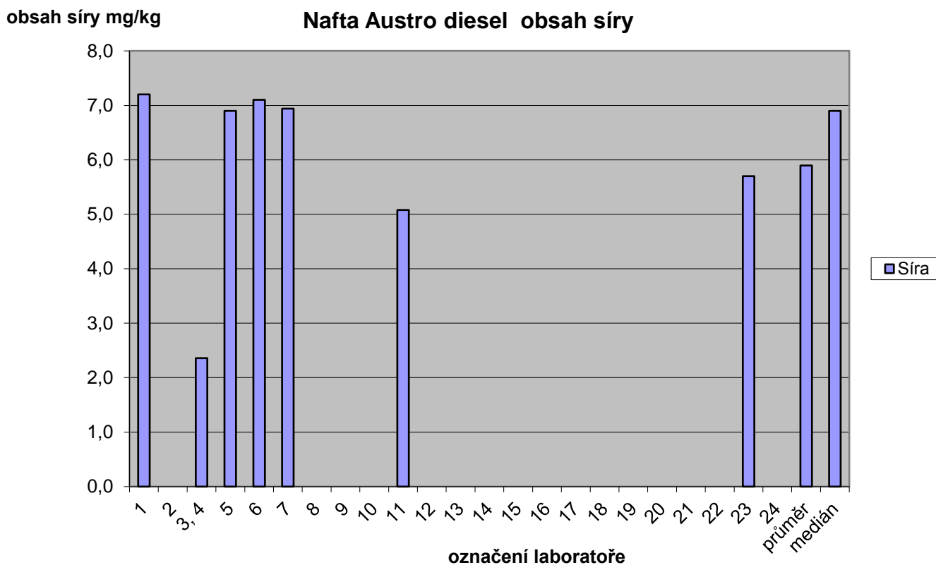
Obr. 7 Obsah síry
