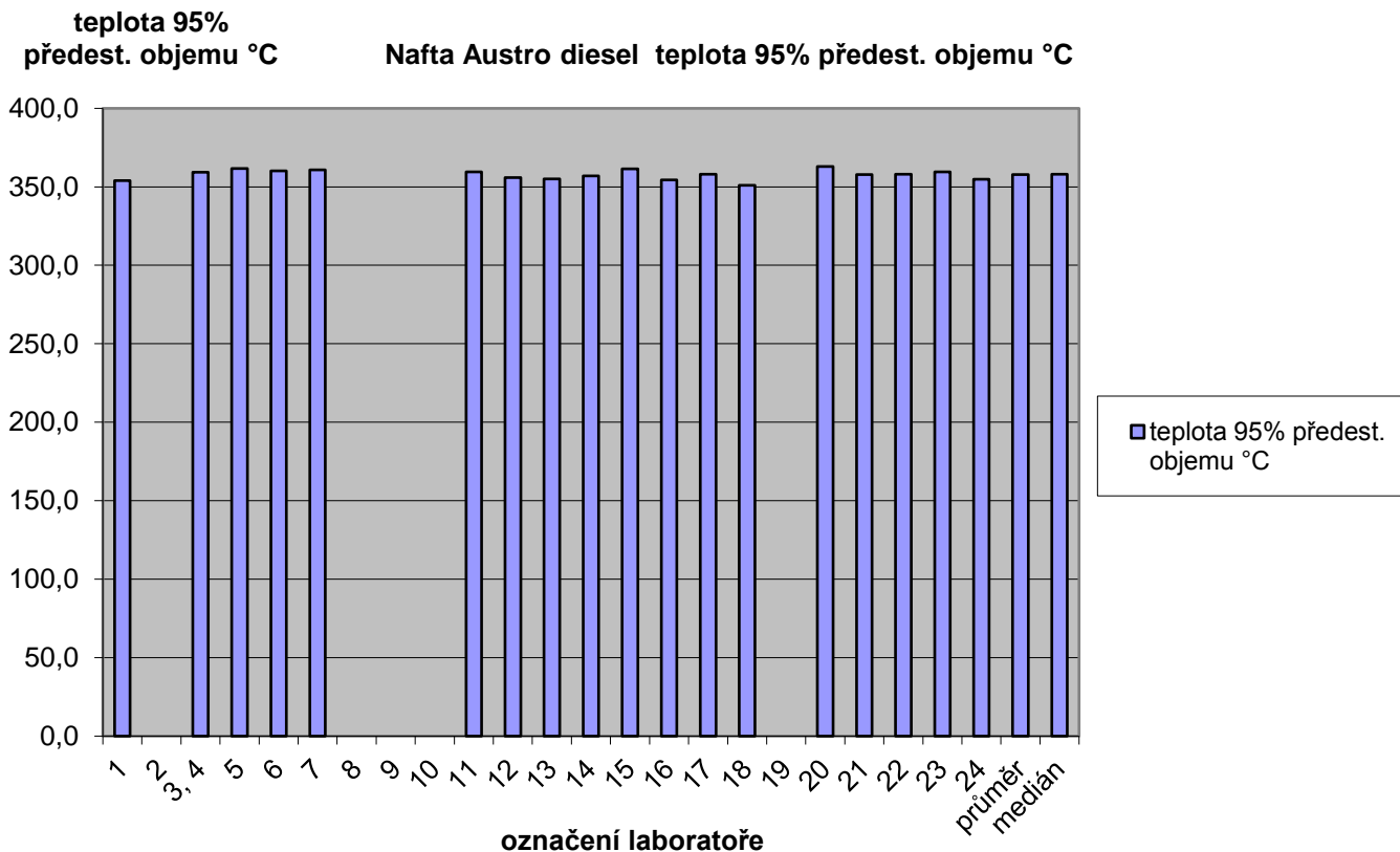
Obr. 4 Destilační zkouška – teplota 95% predest. objemu
