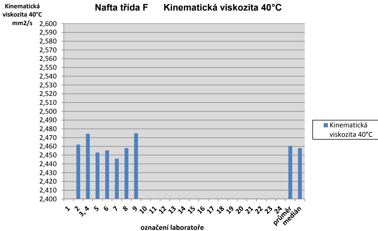
Obr. 16 viskozita při 40°C
