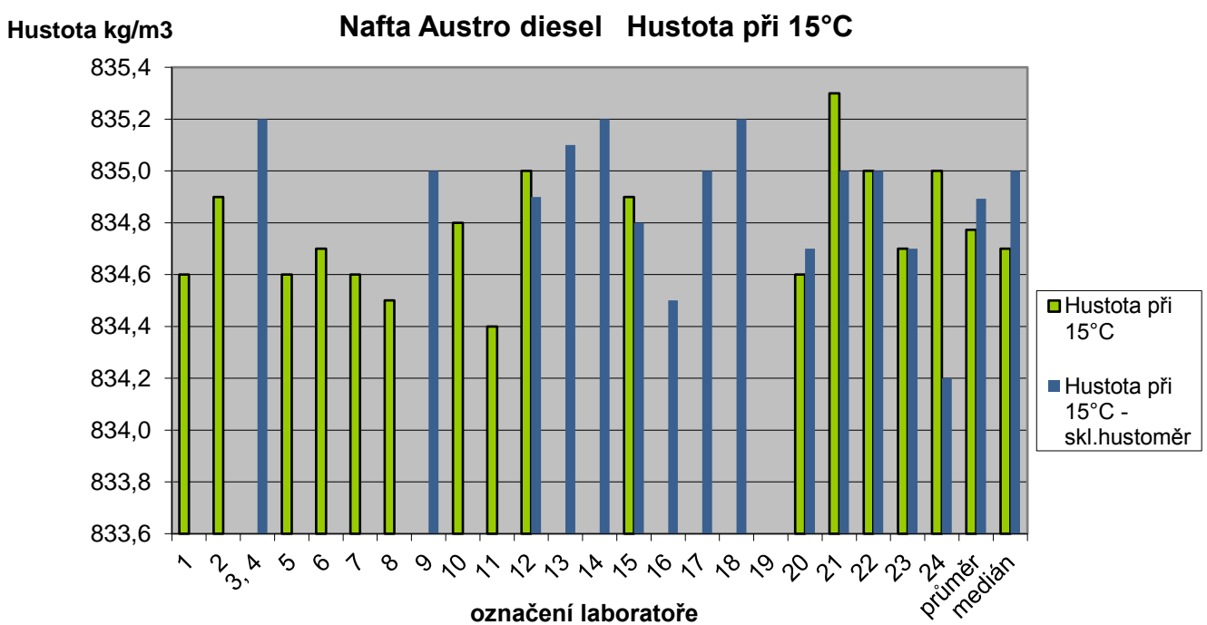
Obr. 2 Hustota 15°C – souhrnné výsledky
