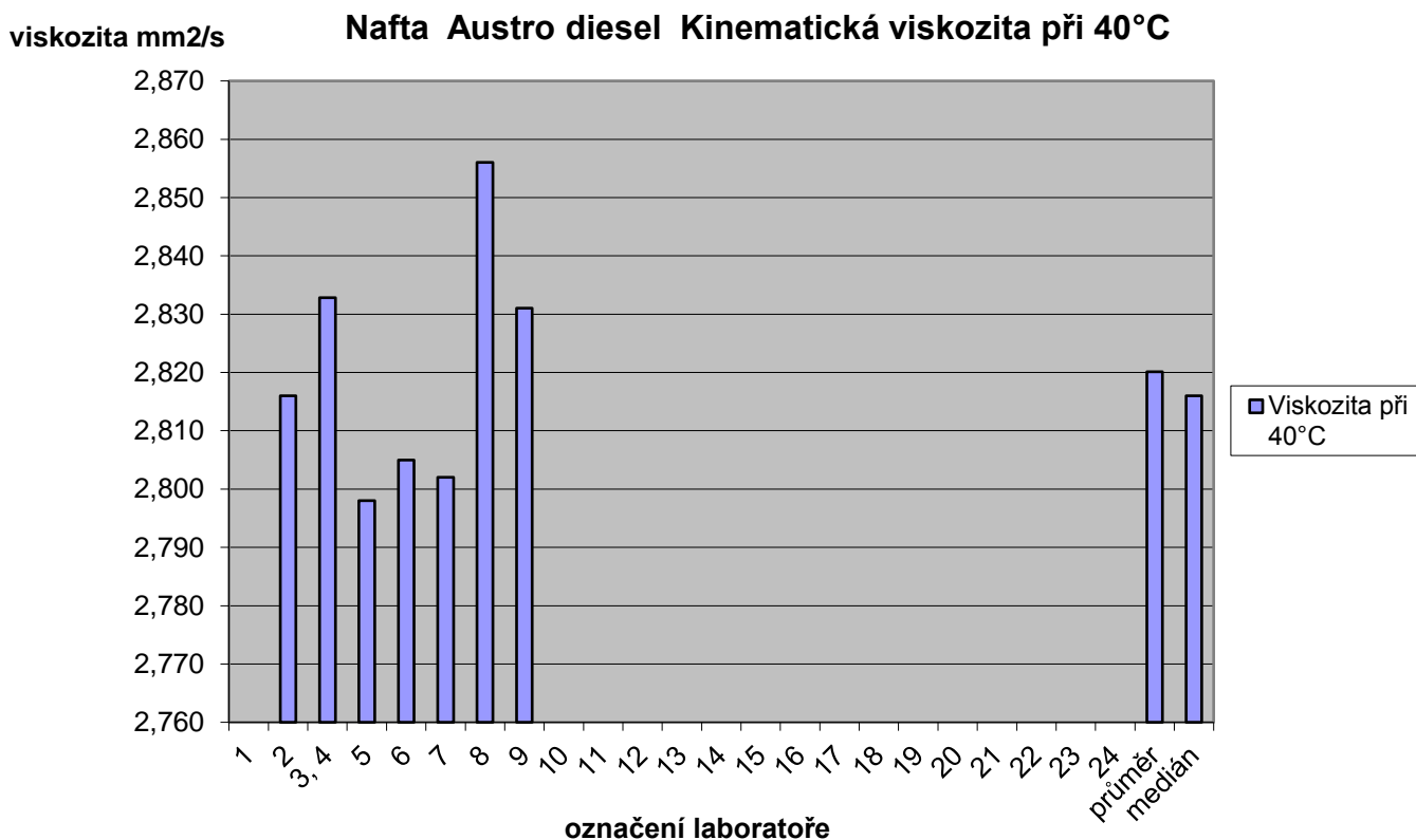
Obr. 8 Viskozita při 40°C
